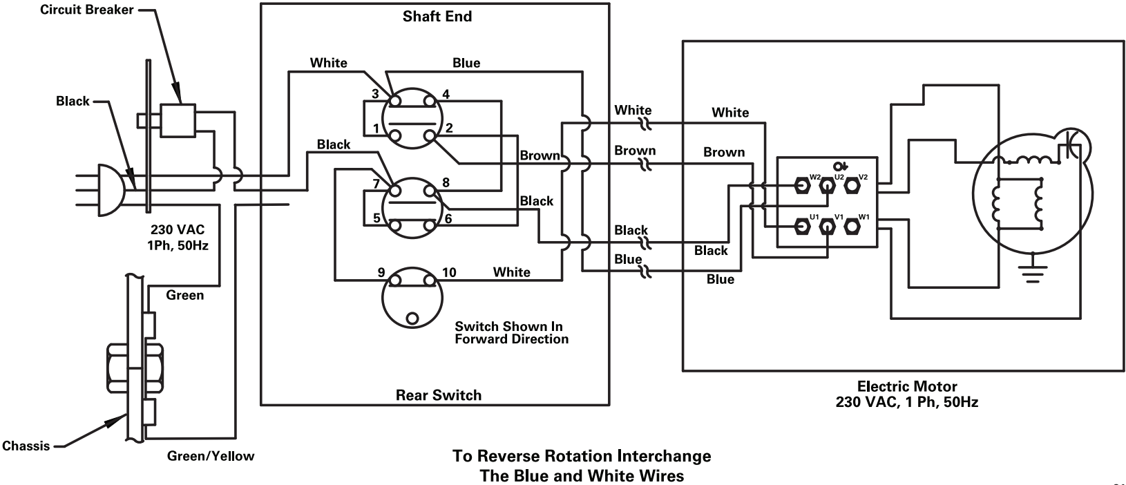
ELECTRICAL DIAGRAM 220 VOLT 50 Hz
